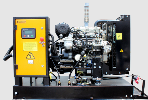
GRUPO ELECTRÓGENO ABIERTO
